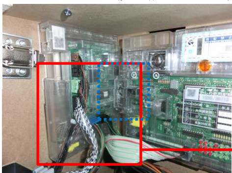
メイン-サブ基板通信ライン全体
