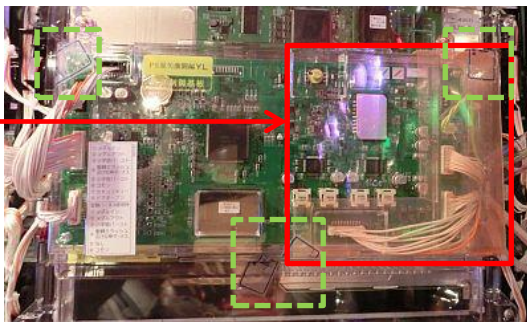
サブ基板側通信ライン対策
