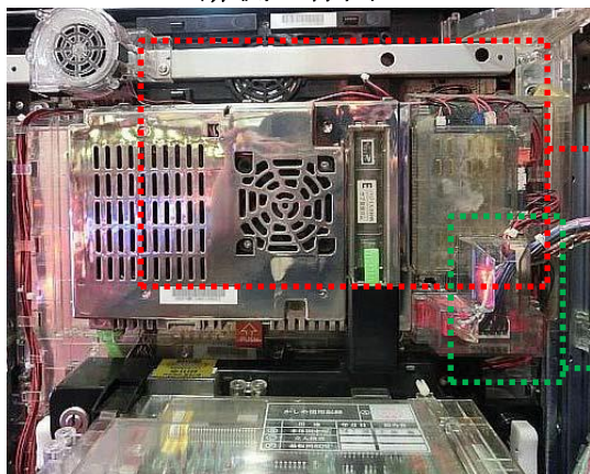
扉側全体図
